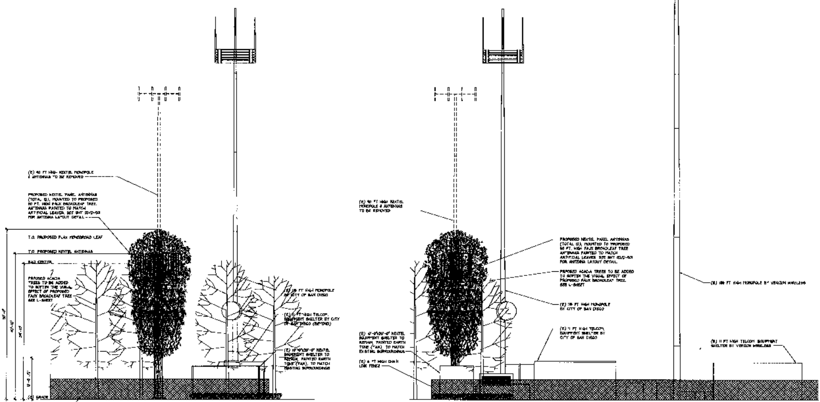
01 NORTH ELEVATION SCALE: 1/8" = 1'-0"
