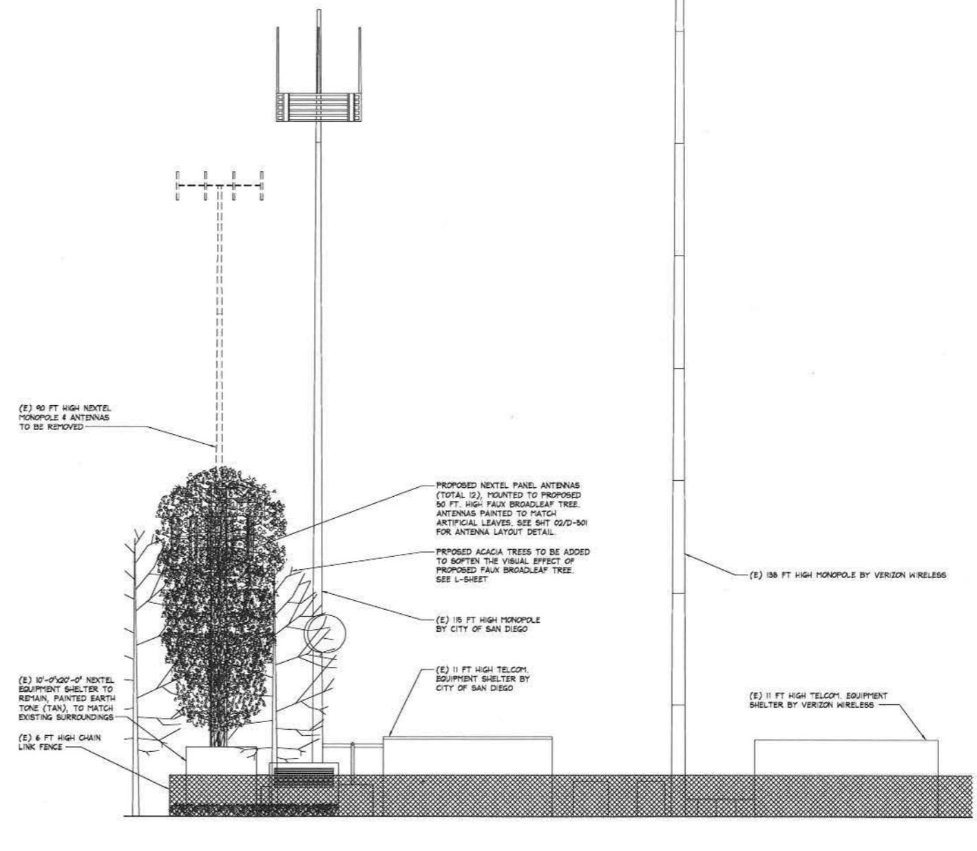
02 WEST ELEVATION SCALE: 1/8" = 1'-0"
