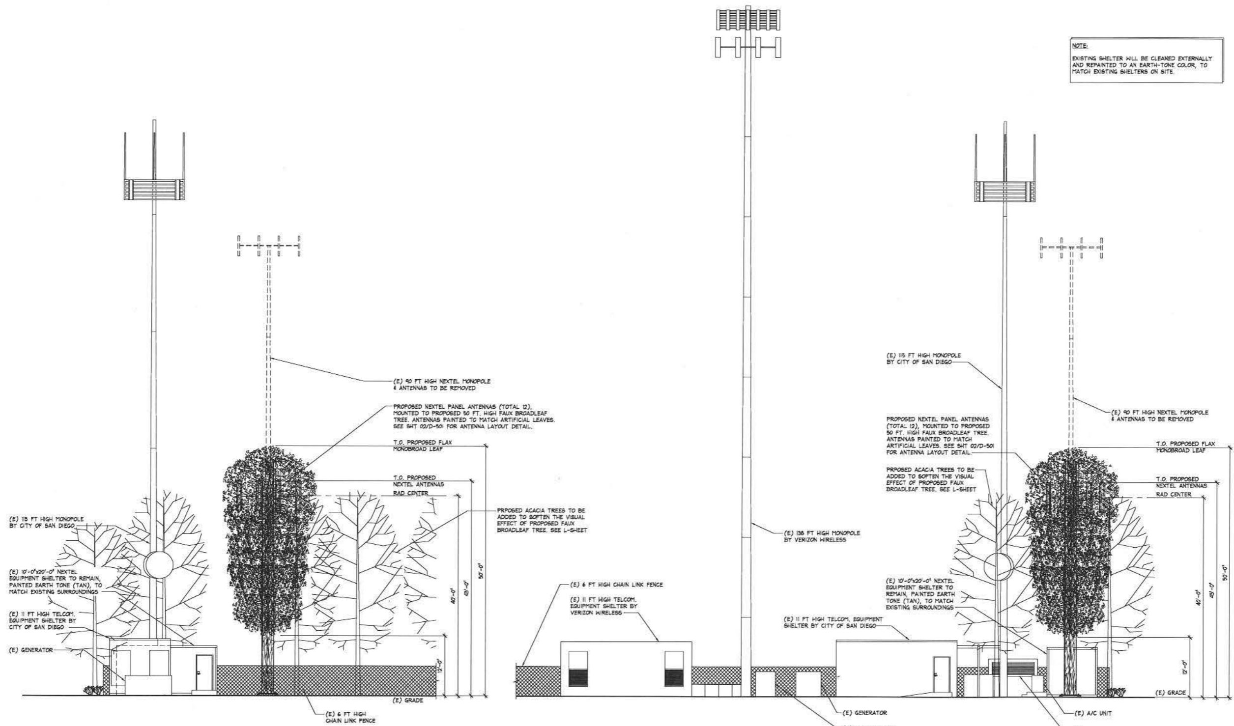
01 SOUTH ELEVATION SCALE: 1/8" = 1'-0"
