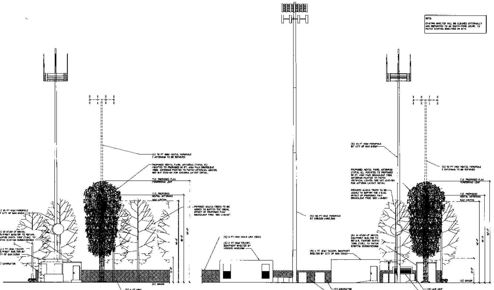
01 SOUTH ELEVATION SCALE: 1/8" = 1'-0"
