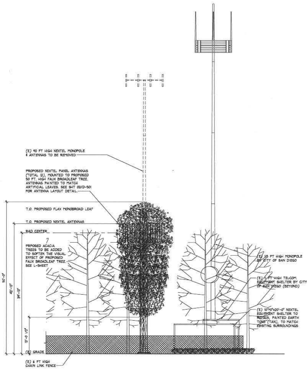
01 NORTH ELEVATION SCALE: 1/8" = 1'-0"
