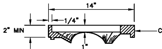
RISER RING
