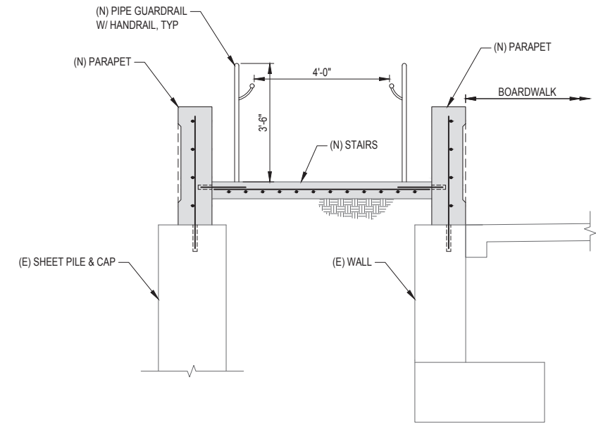
SECTION SCALE: 1/2" = 1'-0"
