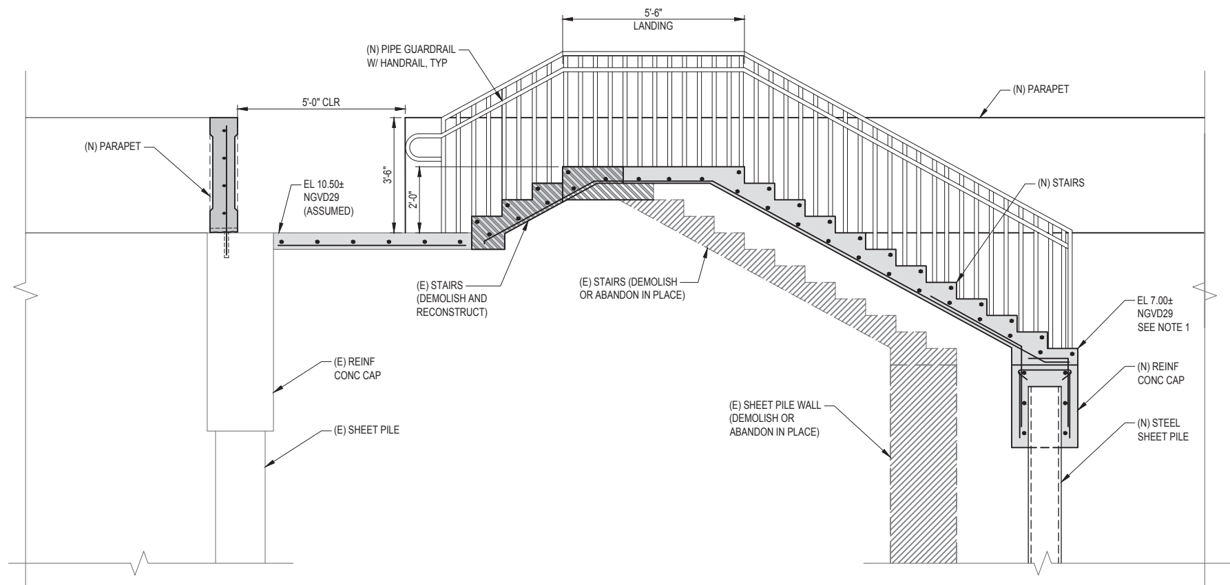
SECTION - STAIRS SCALE: 1/2" = 1'-0"
