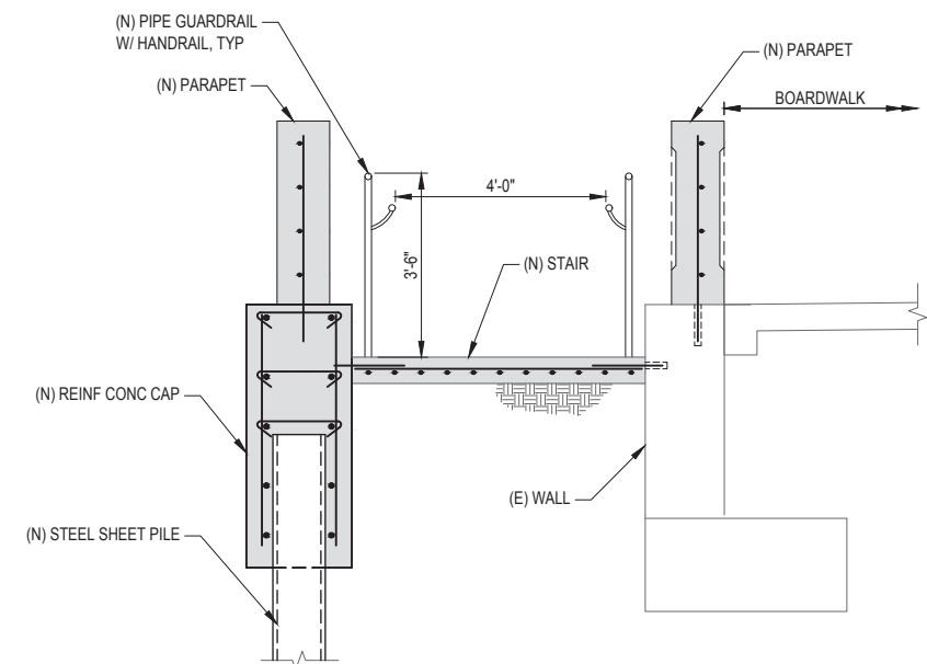
SECTION SCALE: 1/2" = 1'-0"
