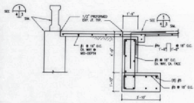
SECTION SCALE: 1/2" = 1'-0"
