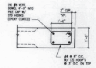
DETAIL SCALE: 1" = 1'-0"
