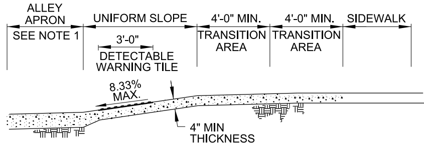
SECTION D-D
